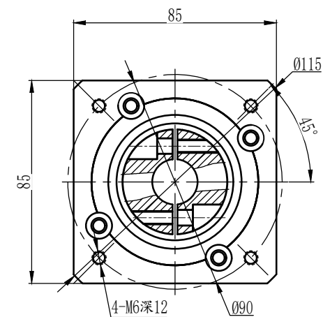
輸入端
