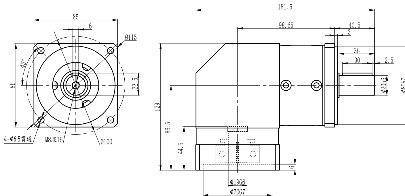
輸出端
