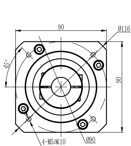
輸入端
